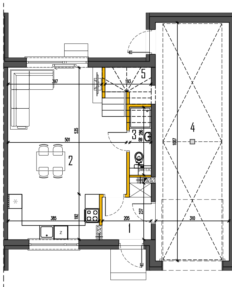
RZUT PARTERU
