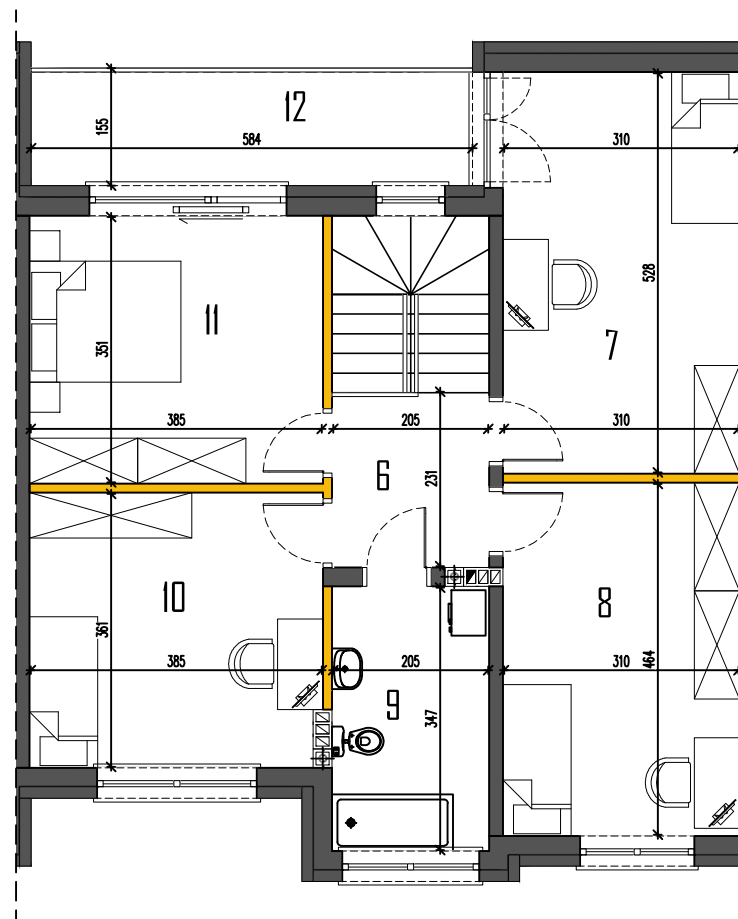
RZUT PIĘTRA
