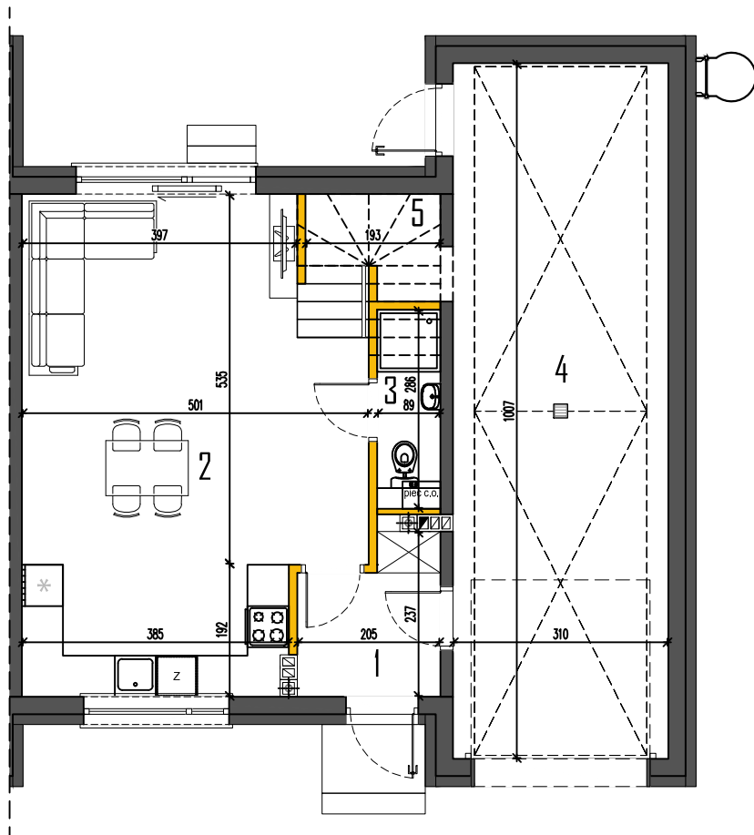
RZUT PARTERU
