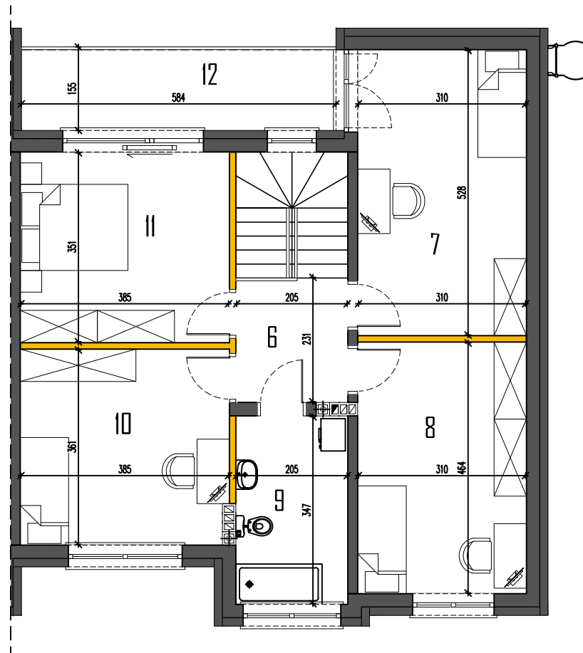
RZUT PIĘTRA
