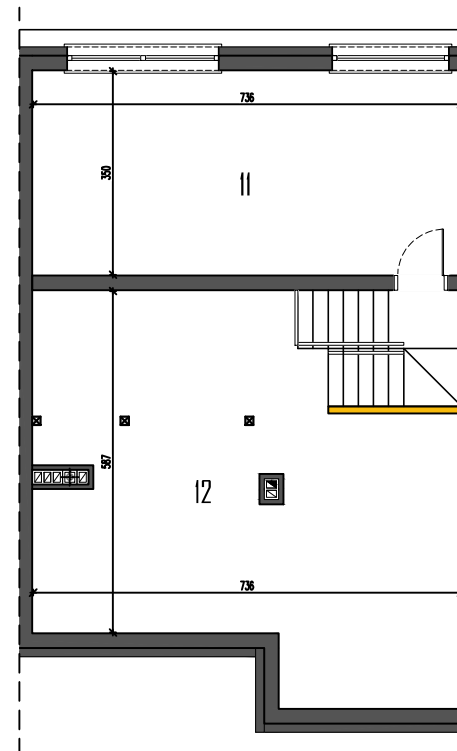
RZUT PÓŁPIĘTRA I PODOASZA
